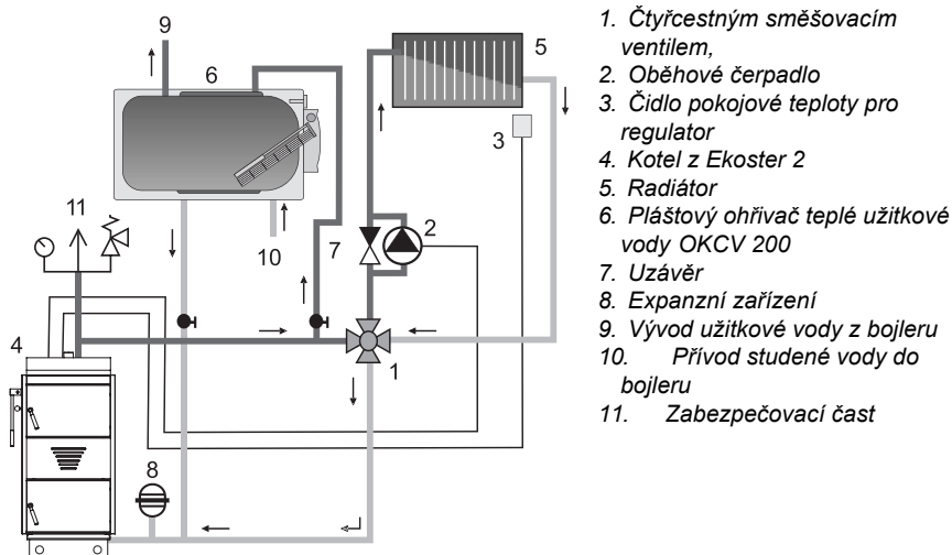
Obr.3 Příklad schéma zapojení kotle Wally Holz se čtyřcestným ventilem a zásobníkem teplé vody
