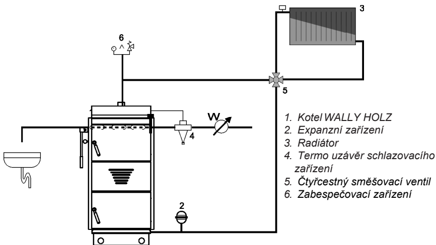
Obr.5 Schéma zapojení termostatického ventilu (např. BVTS) ke kotli Wally Holz
