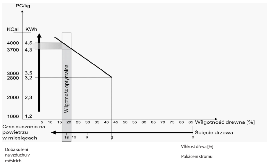
Obr.2 Graf vlhkosti dřeva.
