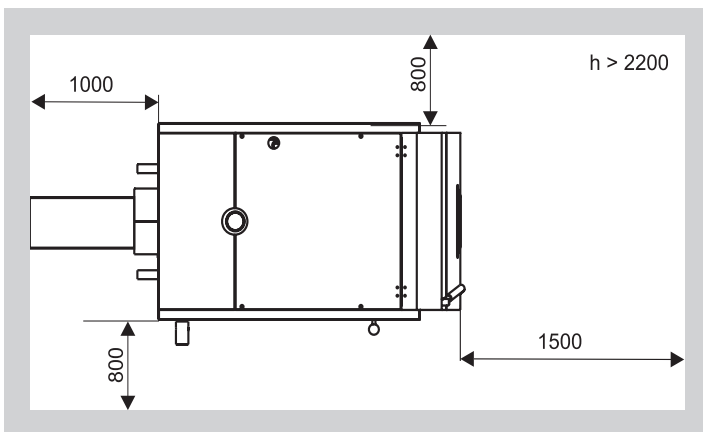
Obr.1 Umístění kotle WALLY HOLZ.
