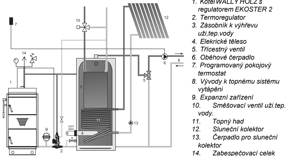
Obr.4 Přiložené schéma systému zapojení vytápění teplé užitkové vody se zásobníkem. S topným hadem a slunečním kolektorem.
